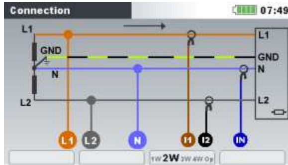
Figure 0.7: Sélection du système 2 phases 4 fils sur l'instrument
