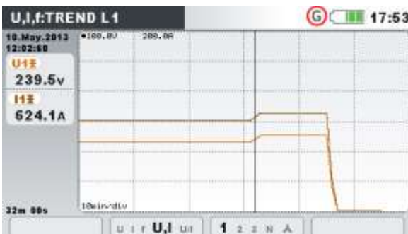
Image 0.18: Tendence de tension et de courant (mode unique)
