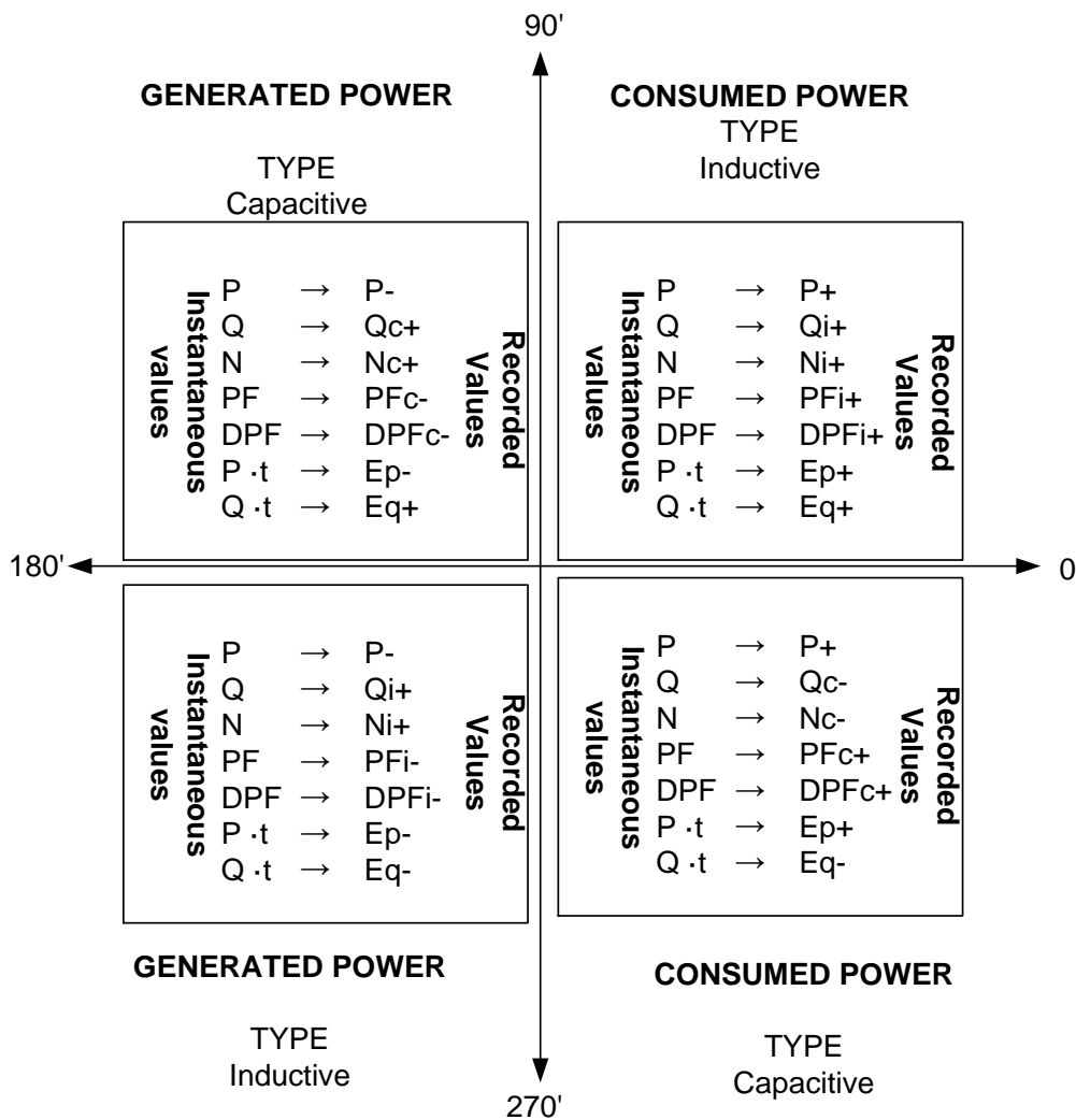
Image 0.11: Diagramme consommée/produite et inductive/capacitive phase/polarité
