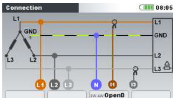
Image 0 : Le choix du système Open Delta (Aaron) à 3 fils sur l'appareil
