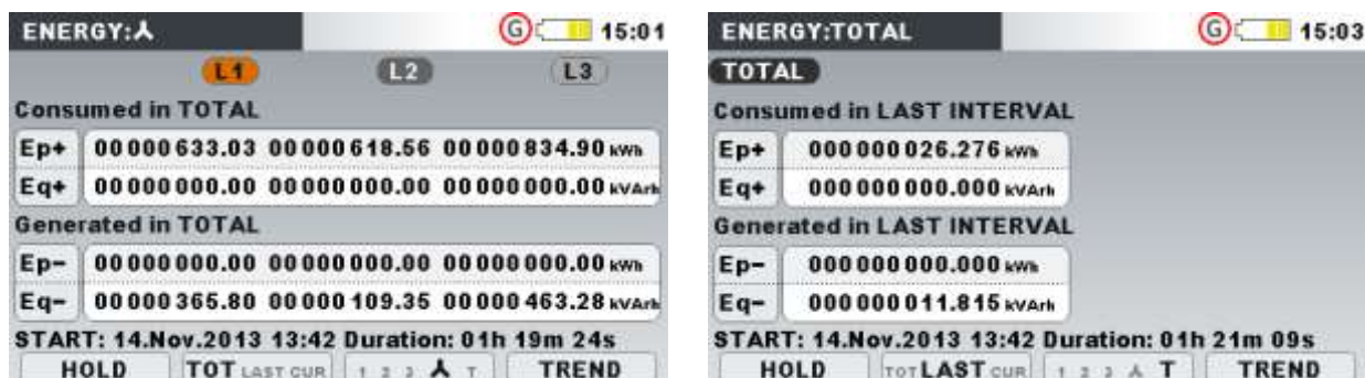
Image0.27: Ecrans des compteurs d'énergie
