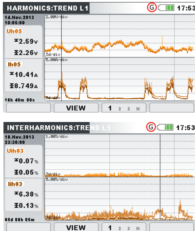
Image0.33: Ecrans de tendance harmoniques et interharmoniques
