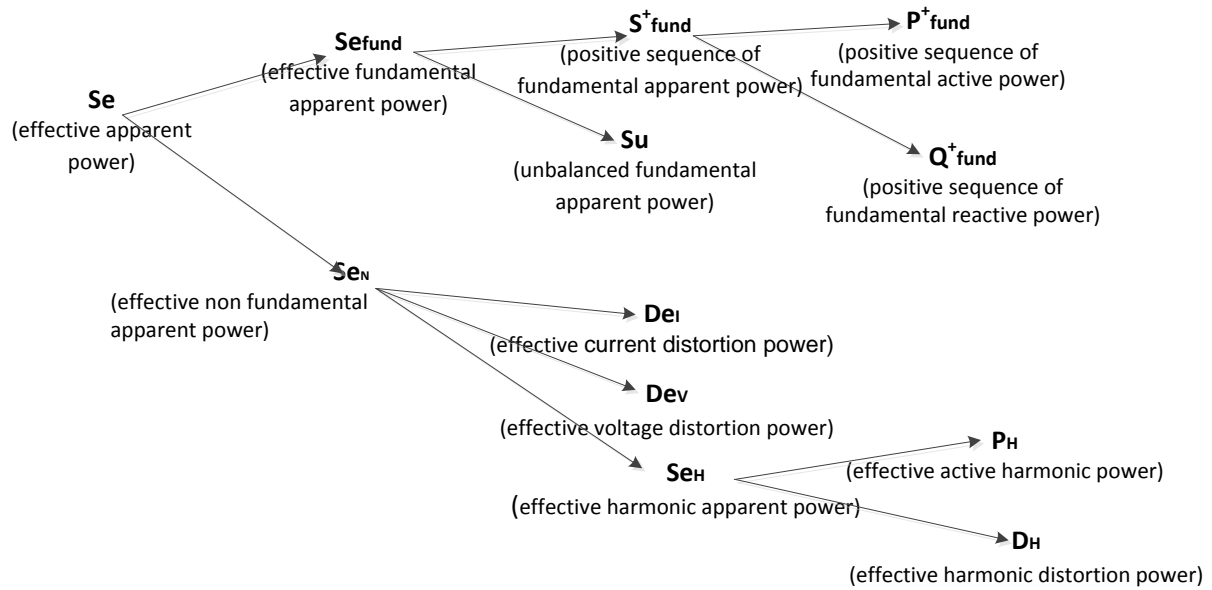
Image 0.3: Organisation de mesure de puissance IEEE 1459 (totaux)
