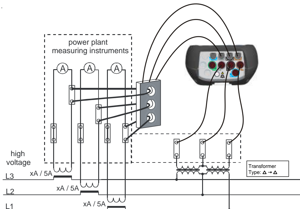
Image0: Connexion de l'appareil aux transformateurs de courant existants dans un système moyenne tension
