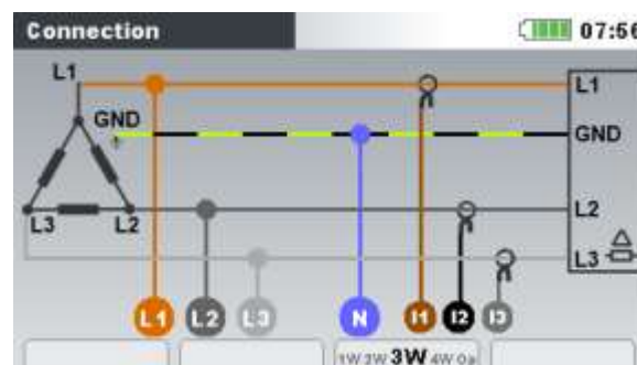
Image 0.5: Choix d'un système triphasé à 3 fils sur l'appareil
