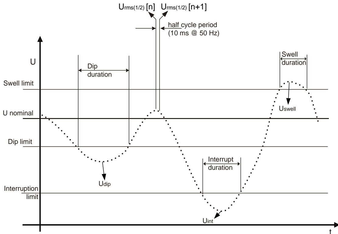
Image 0.9 Définition des événements de tension
