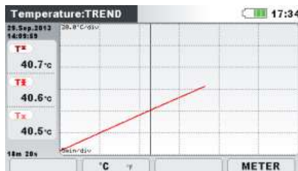
Image 0.40: Ecran de tendance de température
