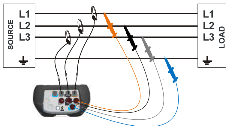
image 0.6: Système triphasé à 3 fils
