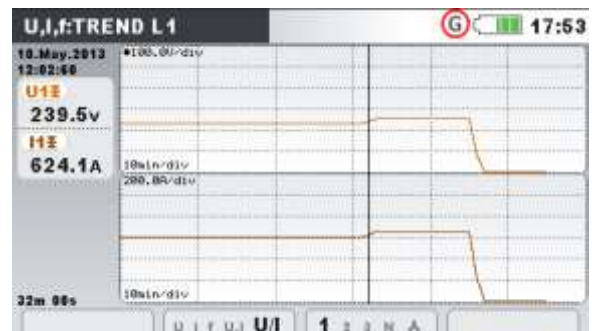
Image 0.19: Tendence de tension et de courant (mode double)
