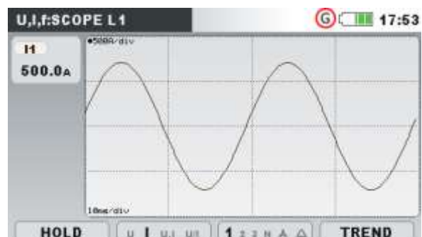
Image 0.13: Forme d'onde unique de courant
