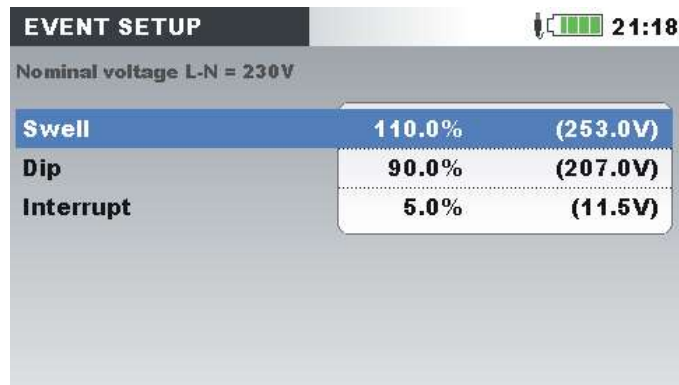
Image3.60: Ecran de configuration d'évènements
