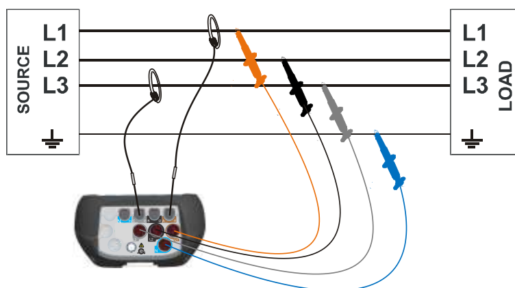
Image 0: Système Open Delta (Aaron) à 3 fils
