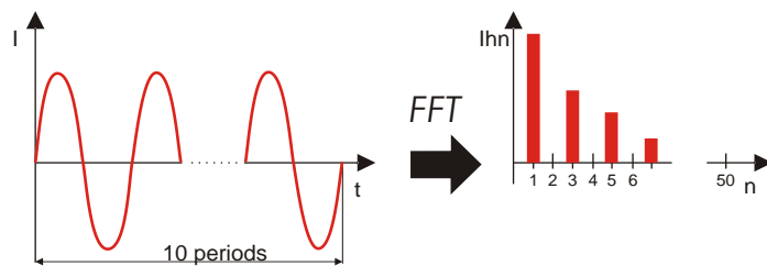
Image 0.6: Harmoniques de courant et de tension
