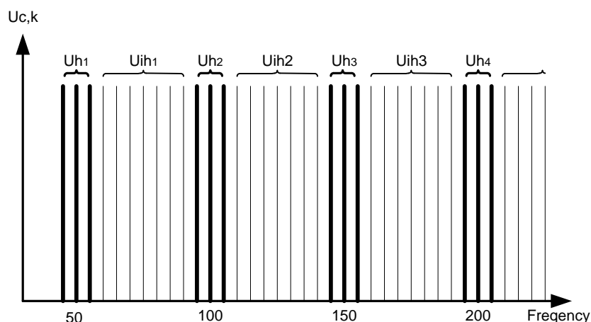
Image0.7: Illustration du sous-groupe d'harmonique pour appareil de 50 Hz
