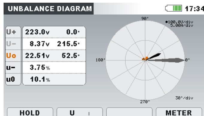
Image0.37: Ecran du digramme déséquilibré
