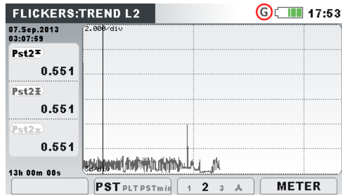
Figure 0.35: Ecran de la tendance du Flickermètre
