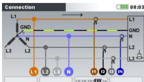
Image0.3: Choisir un système triphasé à 4 fils sur l'appareil
