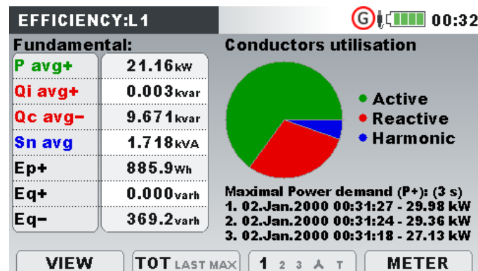
Figure 0.29: Ecran Efficacité Energetique
