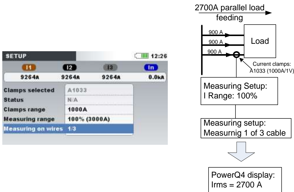
Image0: Distribution parallèle pour les charges importantes
