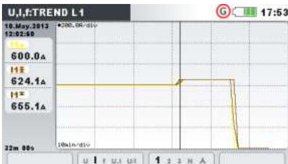
Image 0.20: Tendence de tous les courants
