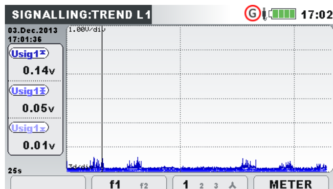
Image 0.44: Ecran de tendance de signalement
