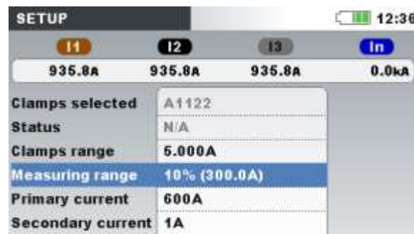
Image 0: Sélection des pinces de courant pour une gamme 10%
