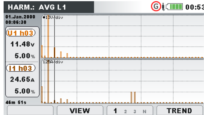
Figure 0.32: Ecran Barregraphes de moyennes d'harmoniques
