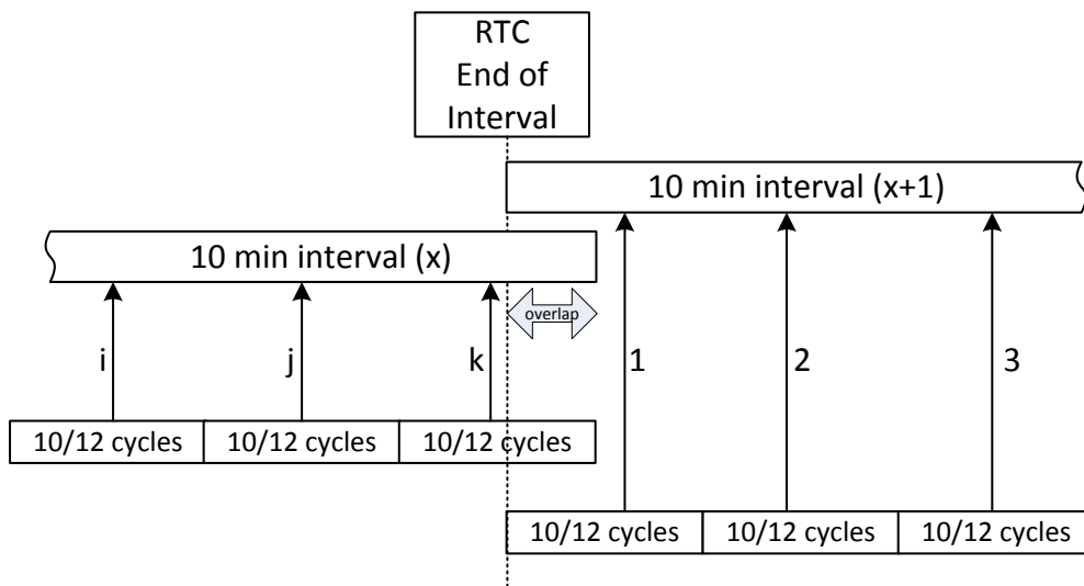
Image 0.110: Synchronisation et regroupement des intervalles de 10 cycles
