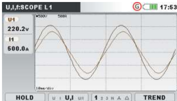
Image 0.14: Formes d'onde de tension et de courant (mode unique)
