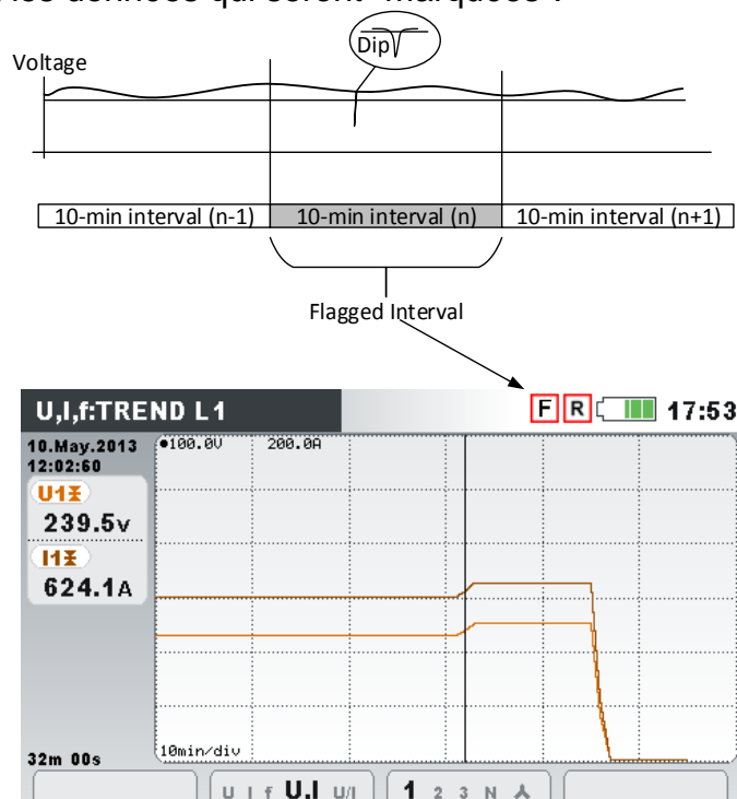
Figure 0.12: Le marquage de données indique que la valeur agrégée peut ne pas être fiable
