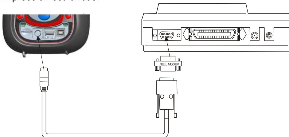
Figure 0.9: Connexion de l'imprimante DPU 414 à l'instrument
