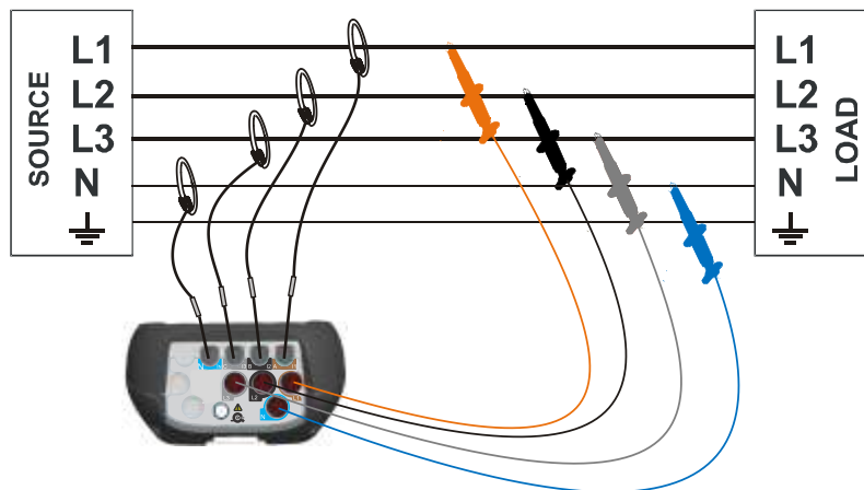
Image 0.4: Système triphasé à 4 fils
