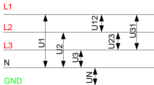
Image 0.1: Tension phase et composée
