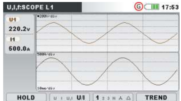
Figure 0.15: Formes d'onde de tension et de courant (mode double)
