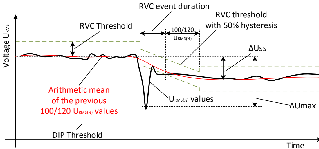
Figure 0.10: Description d'un évènement RVC
