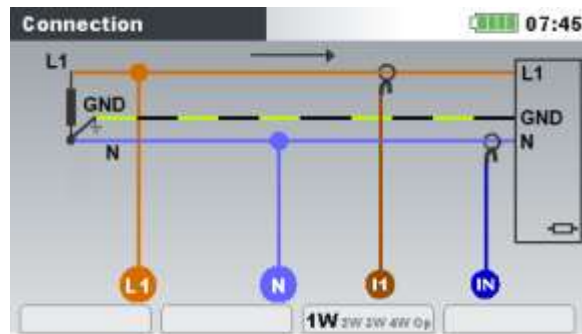
Image0: Le choix d'un système monophasé à 3 fils sur l'appareil
