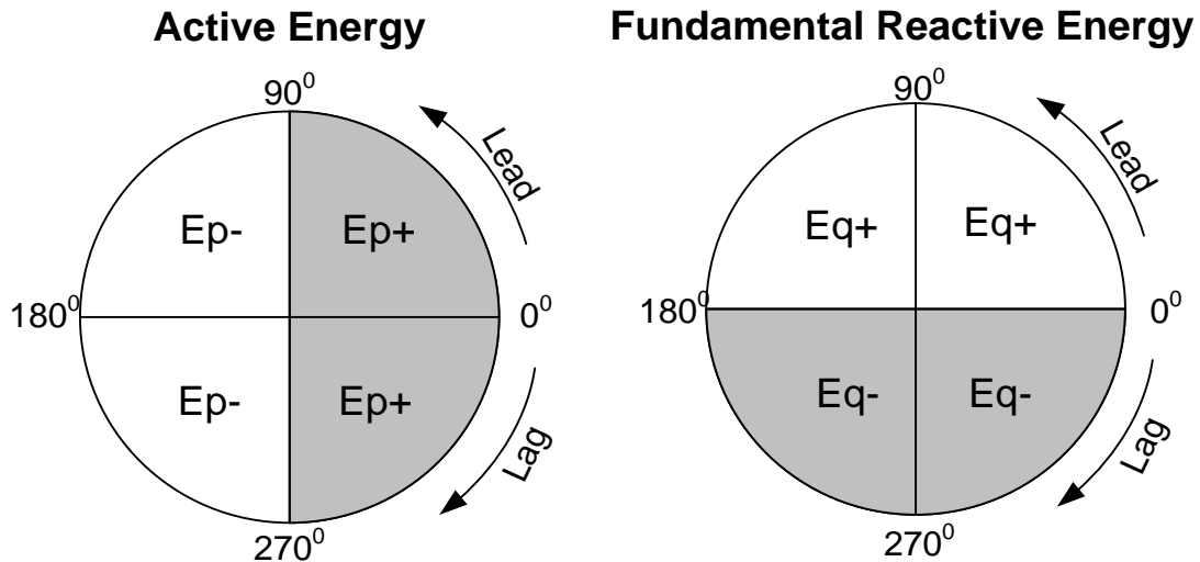
Image 0.4: Relation entre compteurs d'énergie et quadrant
