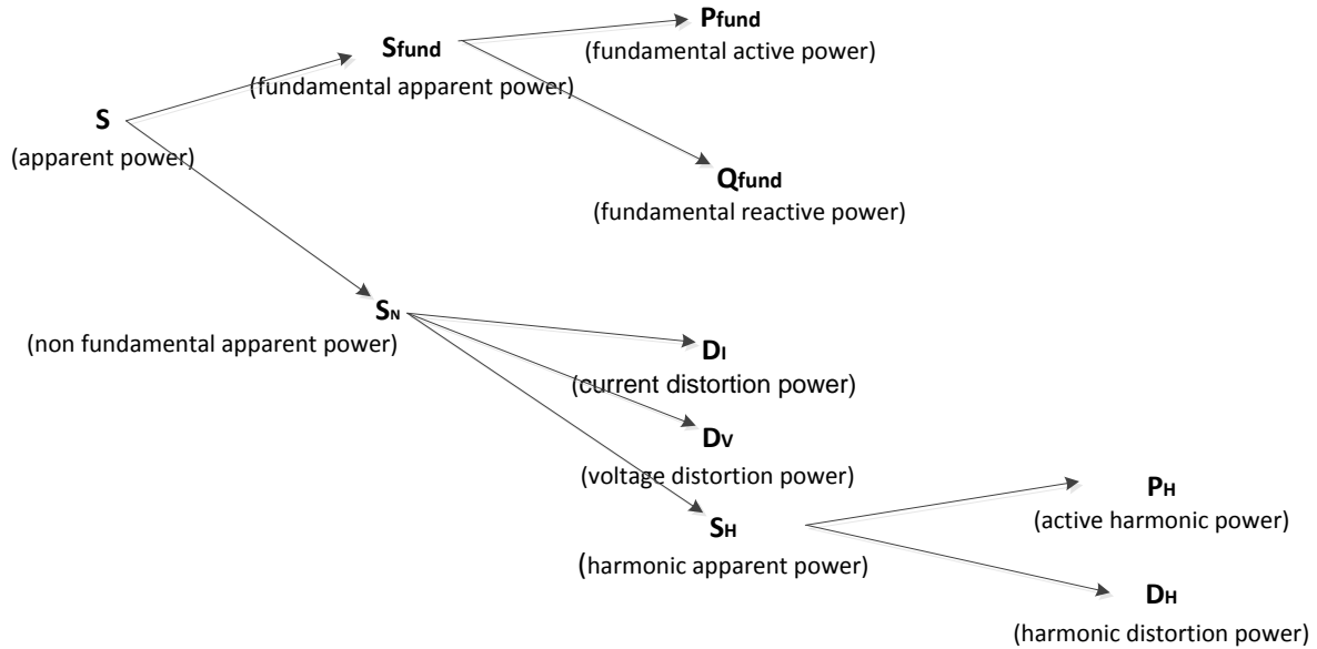
Image 0.2: Organisation de la mesure de puissance de phase IEEE 1459 (phase)
