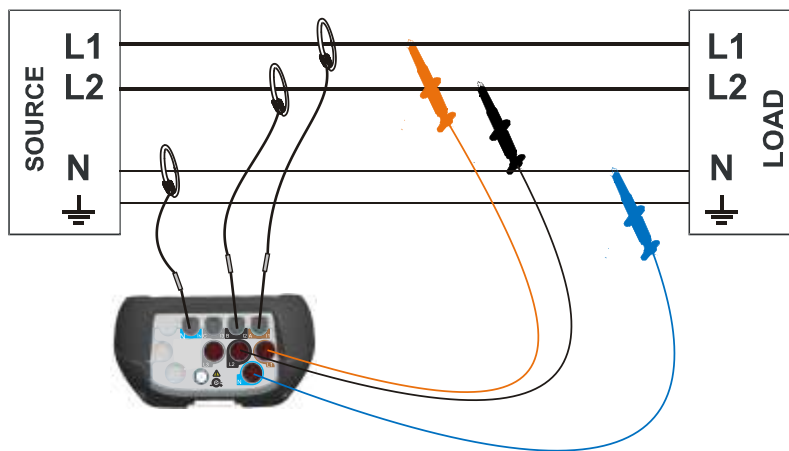
Figure 0.8: Système 2 phases 4 fils
