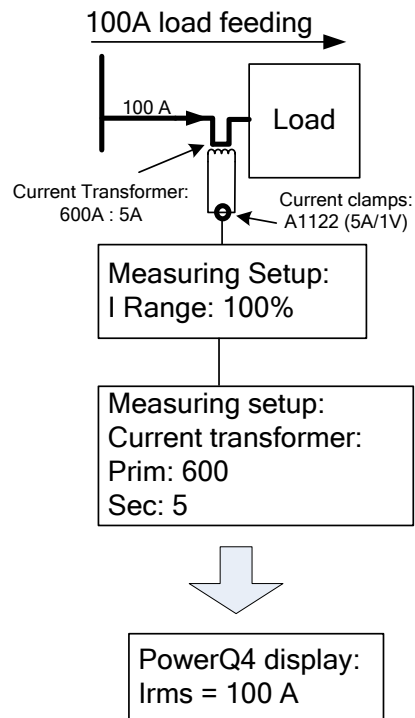
Image0.: Sélection des pinces de courant pour mesure du courant indirecte
