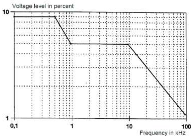
Image 0.17: Niveau limite de tension du réseau de signalment selon la norme EN50160
