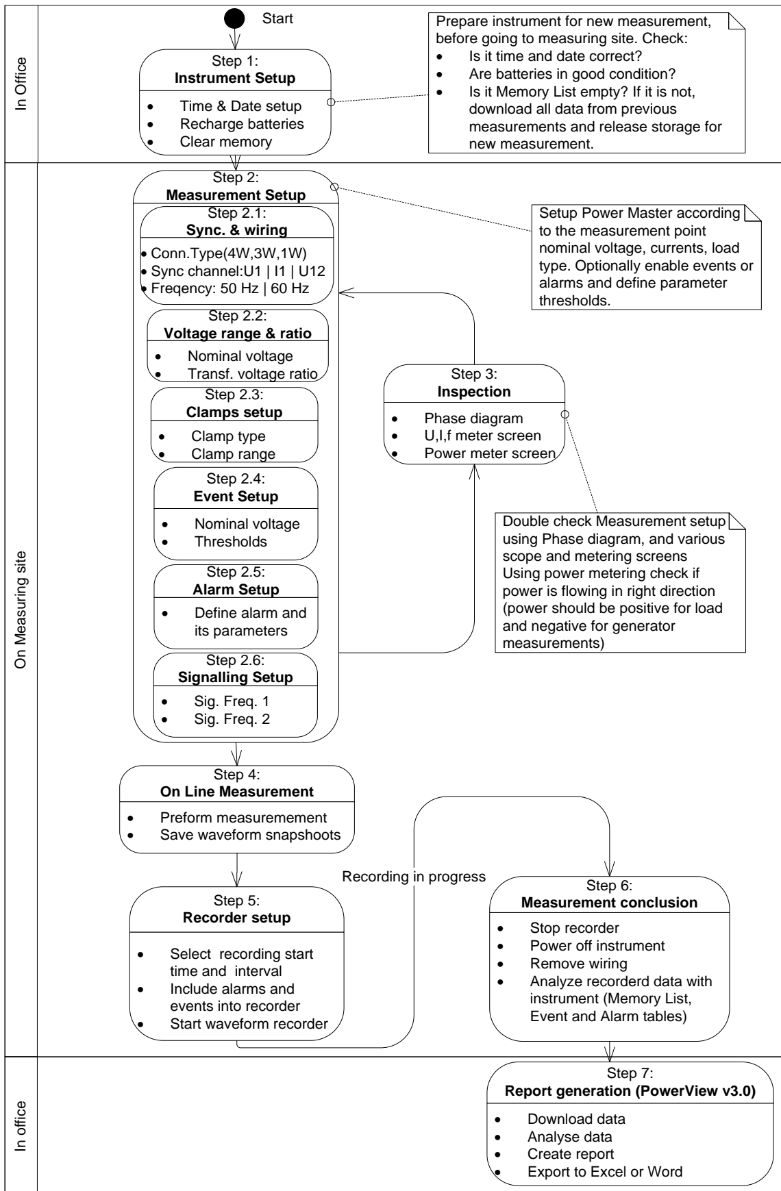
Image 0.1: Procédure de mesure recommandée
