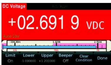
Bargraphe avec mode limite
