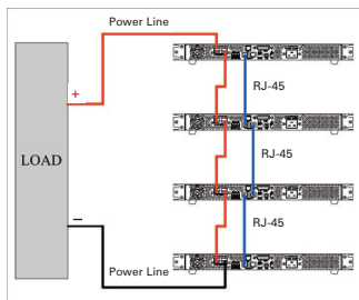
Configuración en Series
