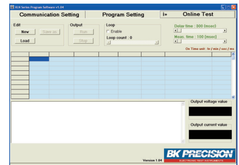
La Prueba Pasa/Falla monitorea los valores de voltaje y de corriente máximos y mínimos sobre un período de tiempo específico
