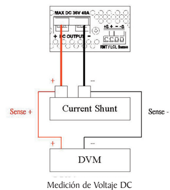
Medición de Voltaje DC
