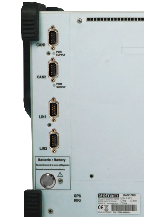
LIN 9 pin D-SUB
